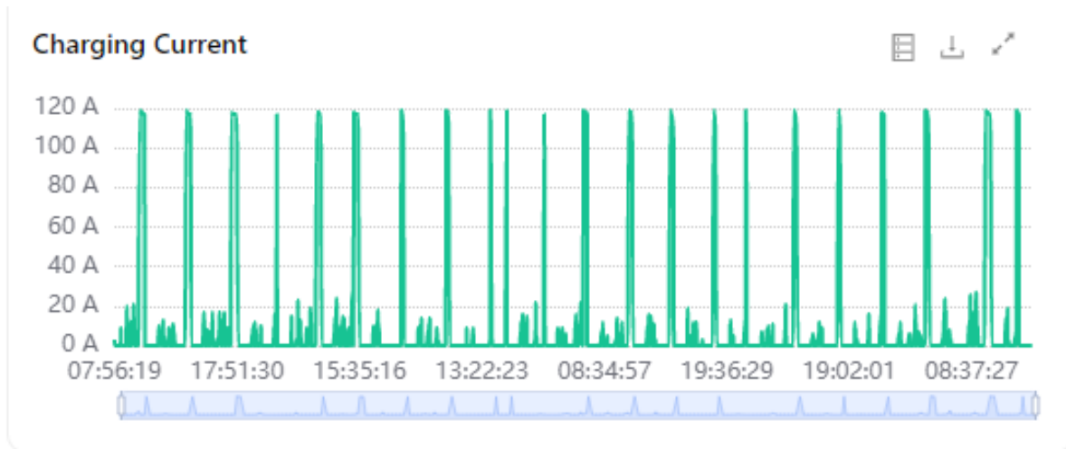
(ウ) バッテリー充電状況 2022/09/12~2022/10/10
